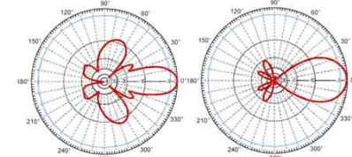
Vertical Horizontal N5 14dBi 안테나 빔 패턴
