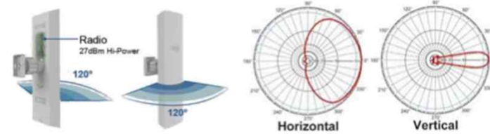
N2S 13dBi 빔 폭 120도 섹터 안테나 빔 패턴
